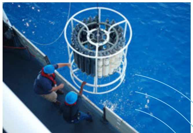
Les prélèvements sont réalisés à partir d'une CDT-rosette © Officiers et équipage du navire PISCES de la NOAA
